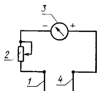
1—платиновый электрод (проволока длиной 50 мм и диаметром 1—2 мм или спираль из нее); 2—переменное сопротивление на 25—50 Ом; 3—милливольтметр типа МПП 254 или милливольт-микроамперметр типов М-95, М-193/2 или другого типа; 4—вольфрамовый электрод (проволока диаметром 0,5—1,0 мм или спираль из нее)
